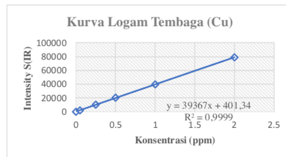
Gambar 2. Kurva Kalibrasi Logam Tembaga (Cu)
