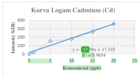
Gambar 3. Kurva Kalibrasi Logam Cadmium (Cd)
