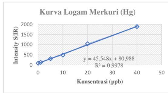
Gambar 1. Kurva Kalibrasi Logam Merkuri (Hg)
