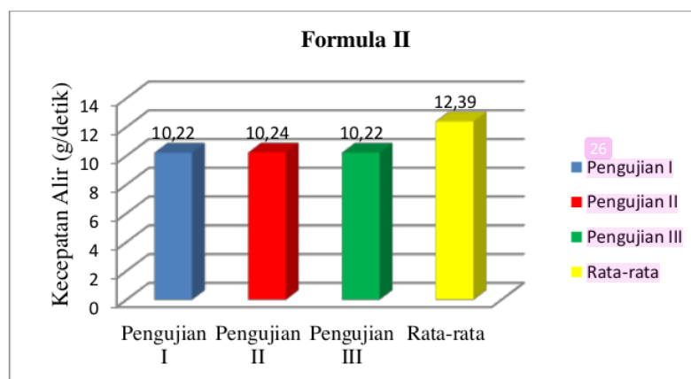
Gambar 2. Hasil pengukuran kecepatan alir formula II
