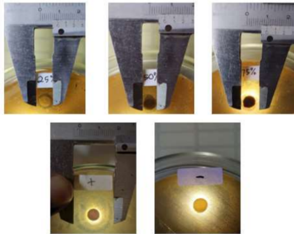
Gambar 2. Hasil penghambatan ekstrak daun sirsak replikasi 1
