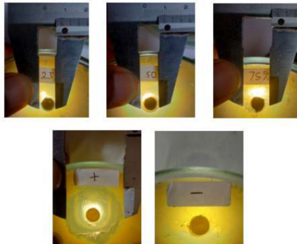
Gambar 3. Hasil penghambatan ekstrak daun sirsak replikasi 2
